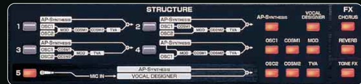
■多彩なシンセサイジング・プロセスをダイレクトに選択できるストラクチャー構成。
